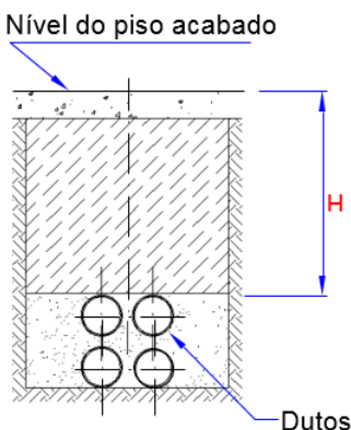
Profundidade de instalação de dutos
